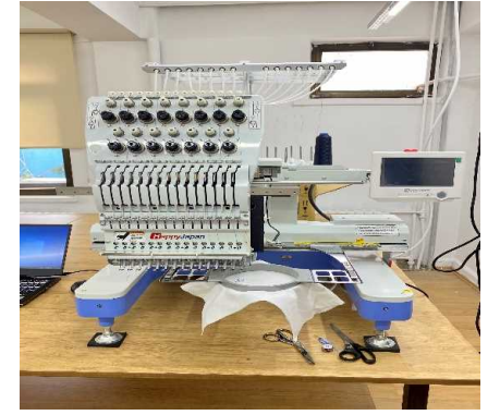
Nakış Makinesi
